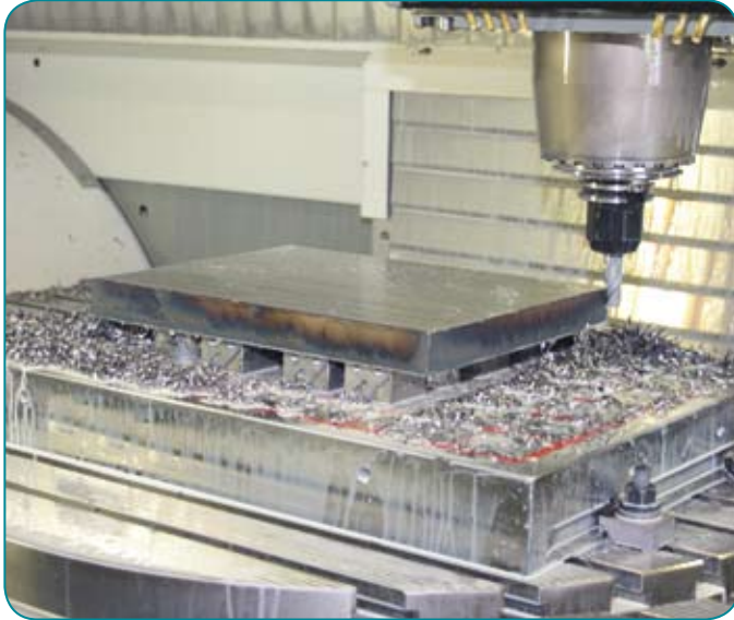
QX HD 70 mit Polverlängerungen für die Bearbeitung von Brennschnitten
