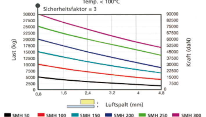
Kraft/Last Luftspalt Kurve auf min. 100mm starkem Stahlblech, vollständig bedeckte Magnetpole. Temp. < 100°C
