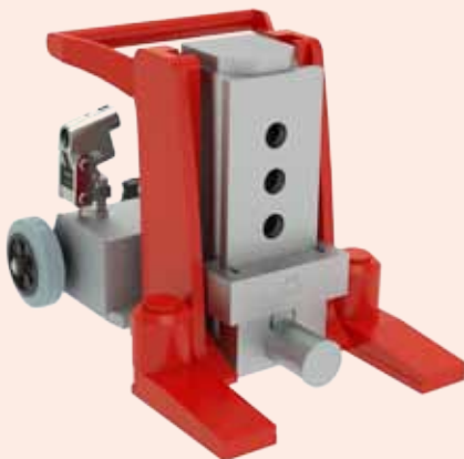
Maschinenheber mit Sonderlasche für Container: die Speziallasche passt in die Containerecken für sicheres Anheben von ISO-Containern, auch nachrüstbar. Erhältlich für alle Heber Serie JH-G plus und JHS 10 ku.
