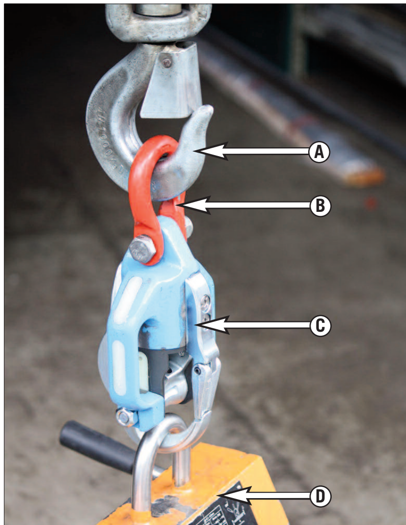
Anschlagart: “Zug über Schäkel/Bohrung”
